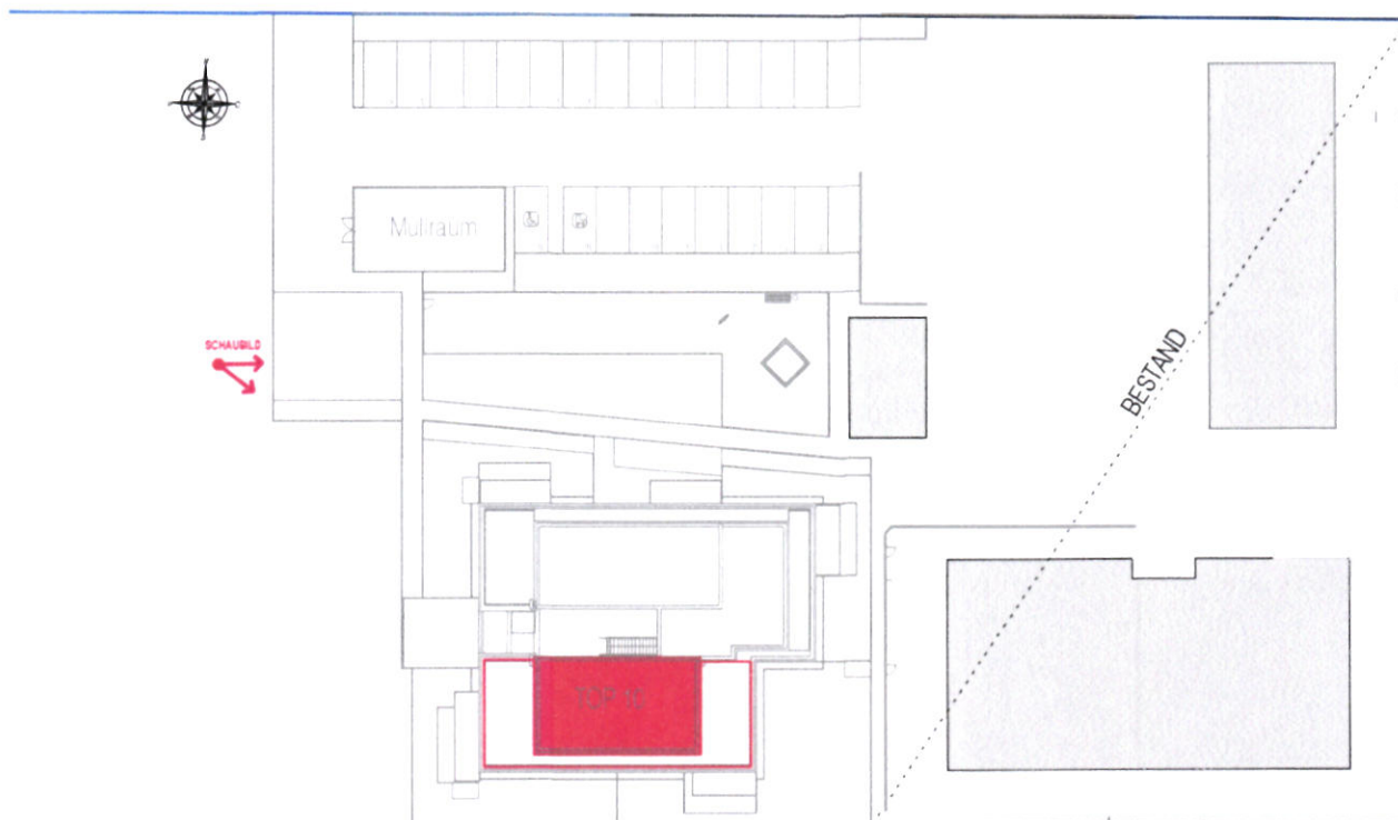
LAGEPLANÜBERSICHT
