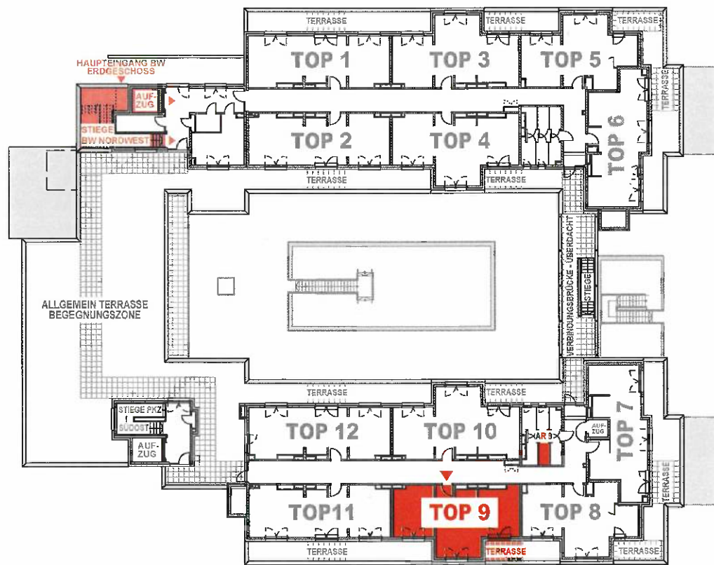
ÜBERSICHTSPLAN - LAGE
